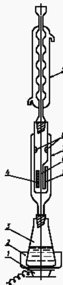
1 — электролитка; 2 — песочная банка; 3 — колба с n -гептаном; 4 — патрон с полимером; 5 — шариковый холодильник; 6 — отверстия; 7 — экстрактор; 8 — ловушка экстрактора; 9 — сифон
